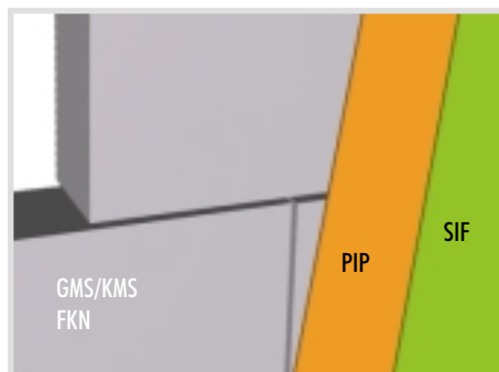
pórobetón - lepený spoj
